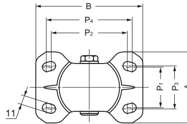
Wheel dia : 100 · 125 · 150mm
