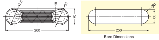
■ APD-KH260
