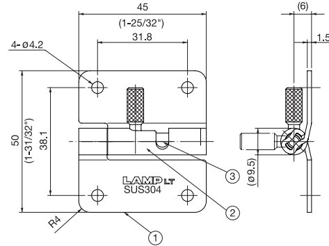
HG-OTA45L
