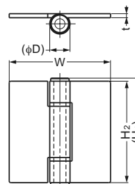
FHS-100
