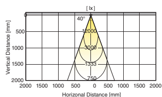
[SL-WPG 3T]
