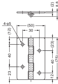
SR75
