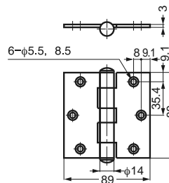
3535SS
