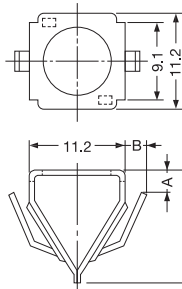
Socket
