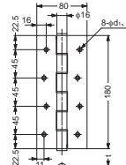
SA 180
