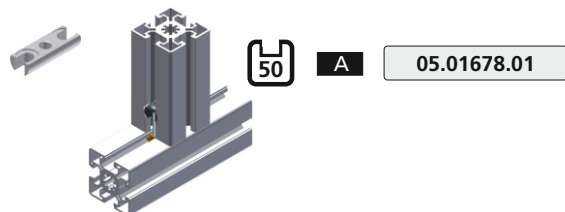
BV Ø17 L=50
