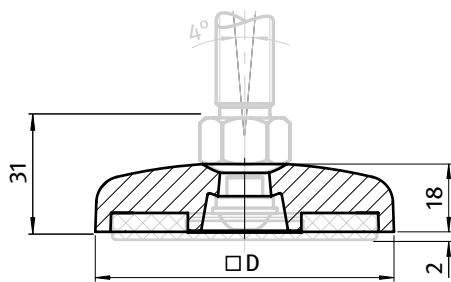
Quadratteller für feste StellfüÙe Square Base for Pivot Feet
