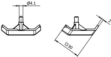
Abdeckkappe 45° Cover Cap 45°
