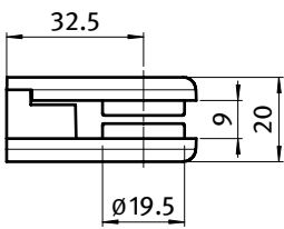
Glasscheibenhalter Glass Panel Clamp
